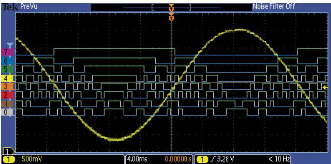
MSO 시리즈는 통합된 16개의 디지털 채널을 제공하여 아날로그와 디지털 신호의 시간상관 관계를 보고 분석하는 데 이용할 수 있습니다.
