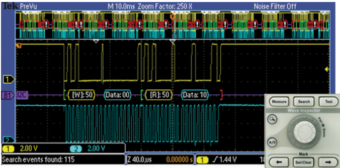
검색 - I°C 디코드는 어드레스 값 50에 대한 Wave Inspector의 결과를 보여 줍니다. Wave Inspector 컨트롤은 파형 데이터를 보고 탐색 기능에서 기대 이상의 효율을 제공합니다.
