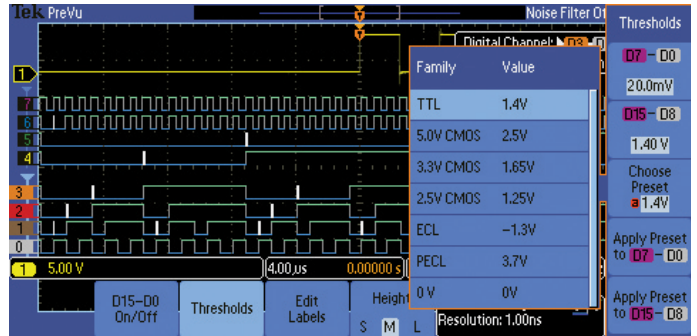
색상으로 코딩된 디지털 파형 디스플레이를 이용하면, 스크린에서 디지털 채널을 설정하여 그룹을 생성할 수 있습니다. 이 경우 디지털 채널은 그룹으로 이동합니다. 8개의 채널의 각 모드에 대한 임계값 설정으로 최대 2개의 다른 로직 패밀리를 지원할 수 있습니다.
