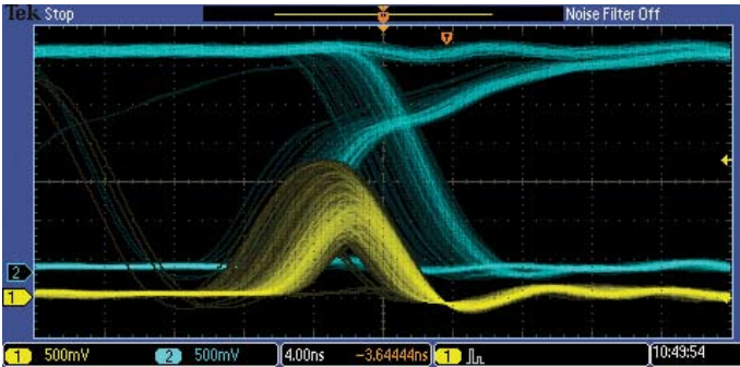
MSO/DPO2000에 적용된 디지털 포스퍼 기술은 5,000 wfm/s 이상의 파형 캡처 속도 및 실시간 명암 그레이딩 성능을 제공합니다.
