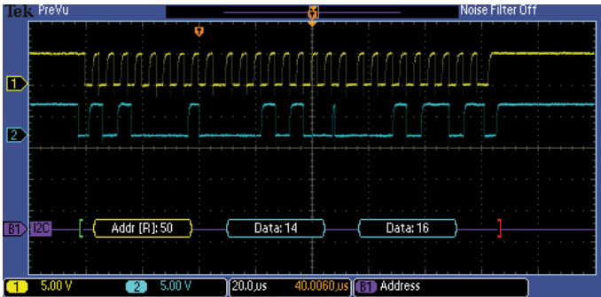
I 2 C 버스 상에서 특정 데이터 패키지에 트리거링. 노란색 파형은 클럭이며 파란색 파형은 데이터임. 버스 파형은 디코딩된 패키지 콘텐츠(Start, Address, Read/Write, Data 및 Stop)를 제공합니다.
