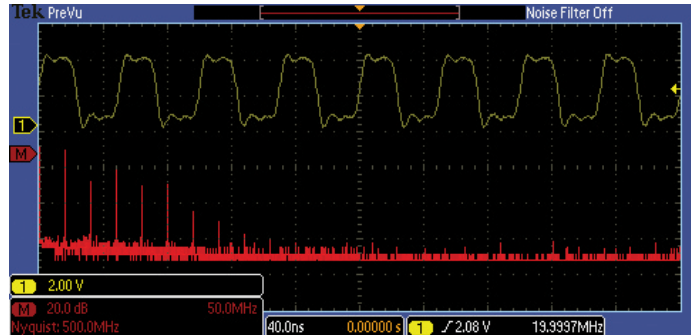
분석 - 펄스 신호의 FFT 통합적인 분석 툴로서 설계의 성능을 빠르게 검증해 줍니다.
