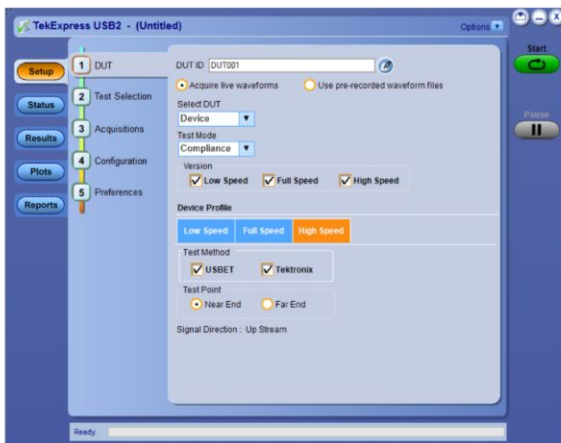
TekExpress USB 2.0 자동 적합성 테스트 구성 메뉴
