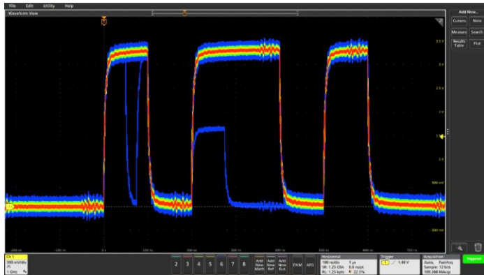
새로운 고해상도 모드와 함께 5 시리즈 MSO의 12 비트 ADC는 업계 최고의 수직 해상도를 가능하게 합니다.
