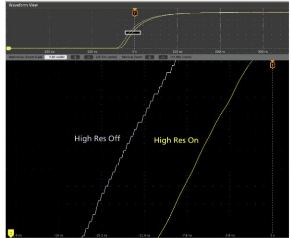
새로운 고해상도 모드와 함께 5 시리즈 MSO의 12 비트 ADC는 업계 최고의 수직 해상도를 가능하게 합니다.
