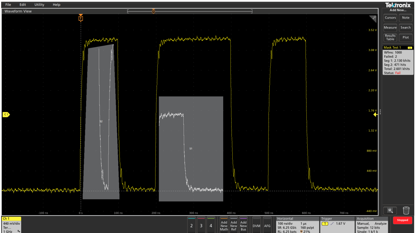
파형의 신호 글리치 및 런트 펄스의 존재를 캡처하는 맞춤형 다중 세그먼트 마스크.
