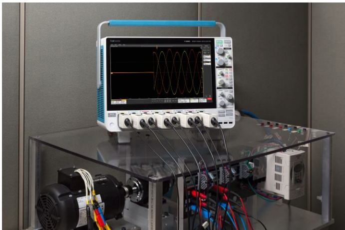
시동 후 3상 입력 전압을 보여주는 3상 모터의 전압 측정.
