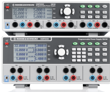
R&S ® HMP2030 3채널 파워 서플라이 R&S ® HMP4040 4채널 파워 서플라이
